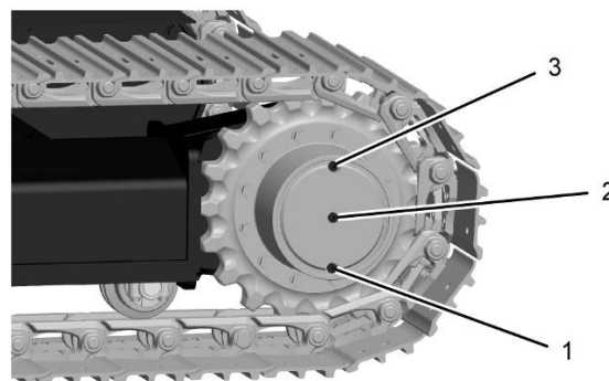
Рисунок 1 (1) Сливная пробка (2) Пробка для контроля уровня масла (3) Пробка маслоналивной горловины
